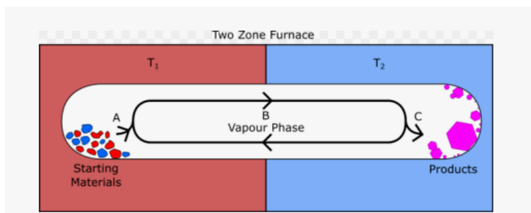
Şəkil2. Kimyəvi nəqliyyat üsullu ilə monokristalın alınması [4]
