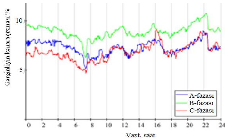
Şəkil 1. Gərginliyin fazalar üzrə kənarlaşması
