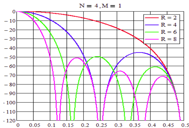
Şəkil 2. Çıxış tezlik reaksiyasının forması
