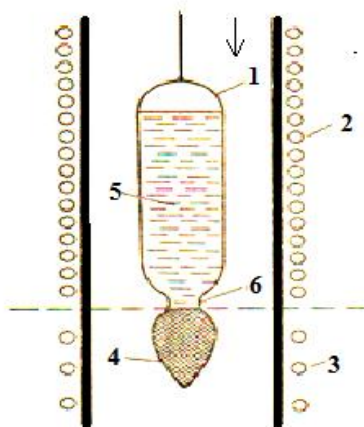
Şəkil1. Bricmen üsulu ilə monokristal yetişdirilməsi qurğusunun sxemi [3]: 1. kvarts ampula 2. Yüksək temperaturlu peç 3. Aşağı temperaturlu peç 4. dar hissə 5. Kristallaşan maddə
