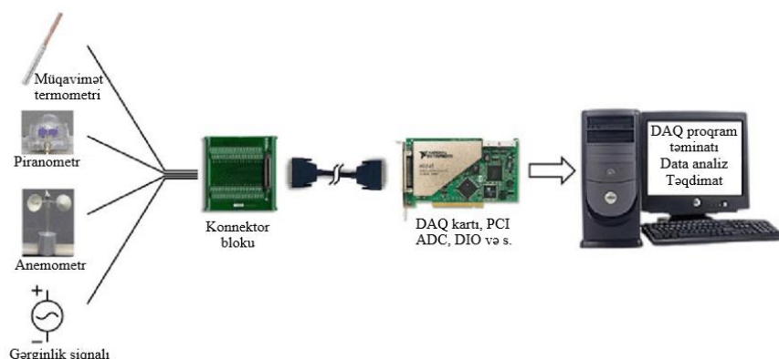
Şəkil 2. Nəzarət-idarəetmə sistemi
