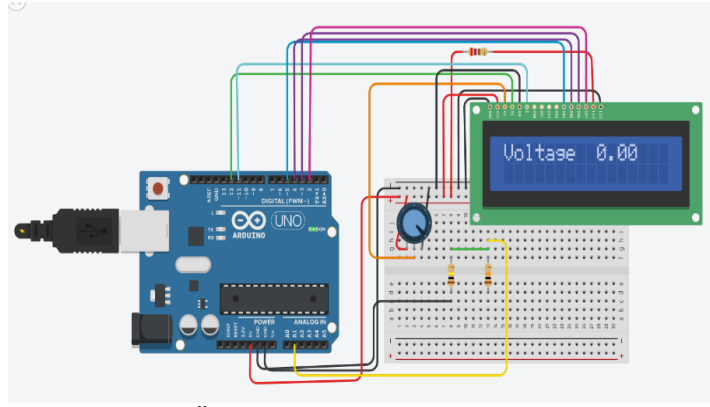
Şəkil 1. Ölçü cihazının simulyasiya variantı
