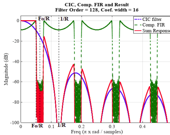
Şəkil 2. Təshihedici süzgəcin tezlik reaksiyası və parametrləri
